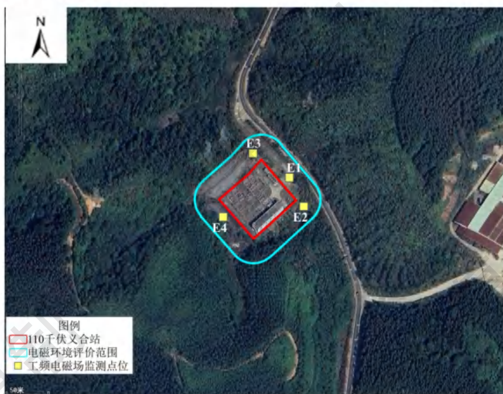
图 1 本工程测量布点图
