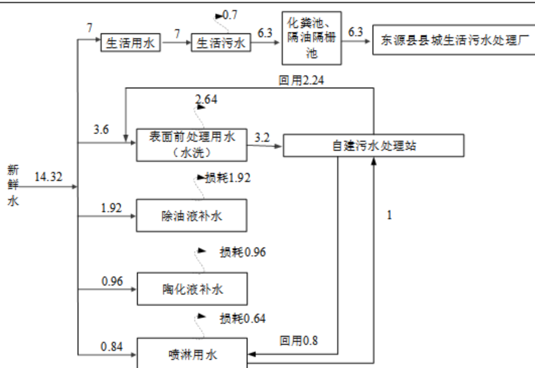
图 2-1 扩建项目水平衡图 \text{m}^3/\text{d}
