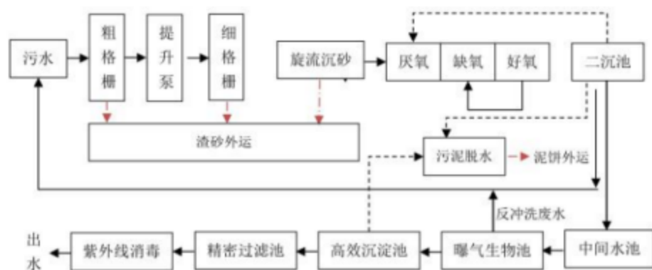
图 4-2 东源县城污水处理厂一期处理工艺流程图
