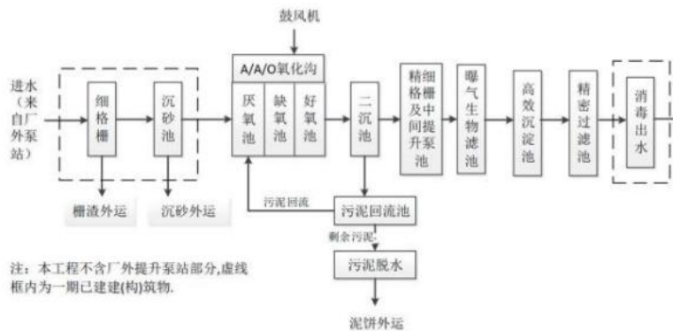
图 4-3 东源县城污水处理厂二期处理工艺流程图
