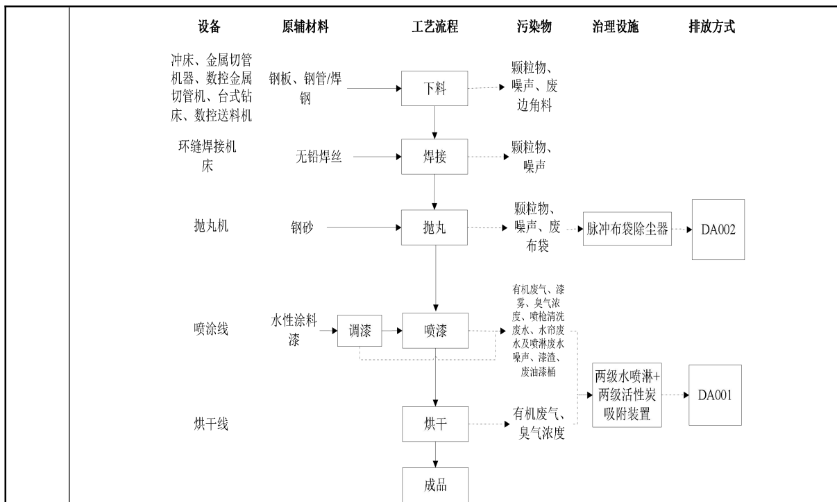
图 2-5 钢制脚手架工艺流程及产污环节示意图
