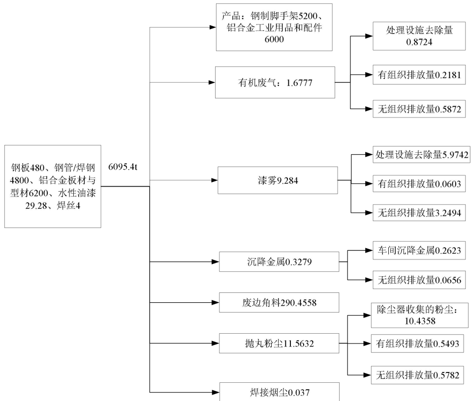
图 2-3 项目物料平衡图 (t/a)
