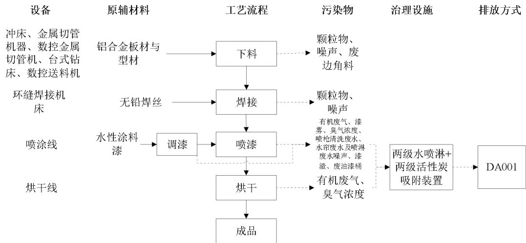
图 2-6 铝合金工业用品和配件工艺流程及产污环节示意图
