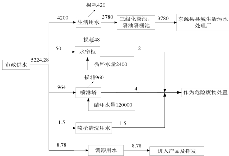
图 2-2 项目水平衡图 (单位 m³/a)
