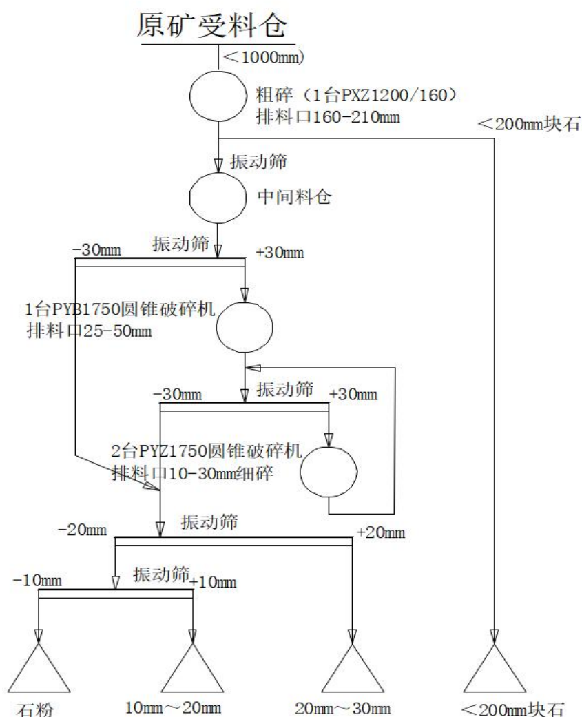
图 6-1 破碎加工工艺流程图
