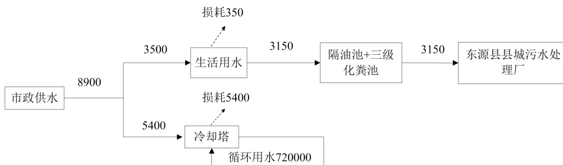
图2-3 改扩建后全厂水平衡图 (单位m³/a)
