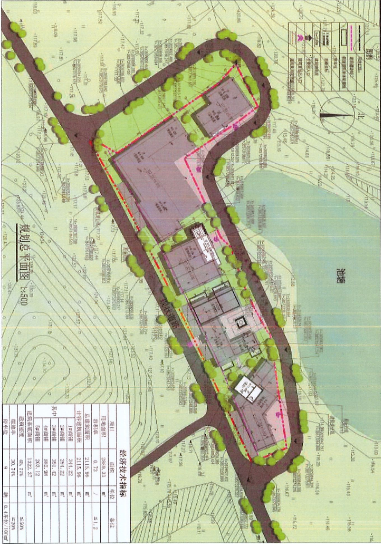
彩色总平面图 Color General Layout Plan
