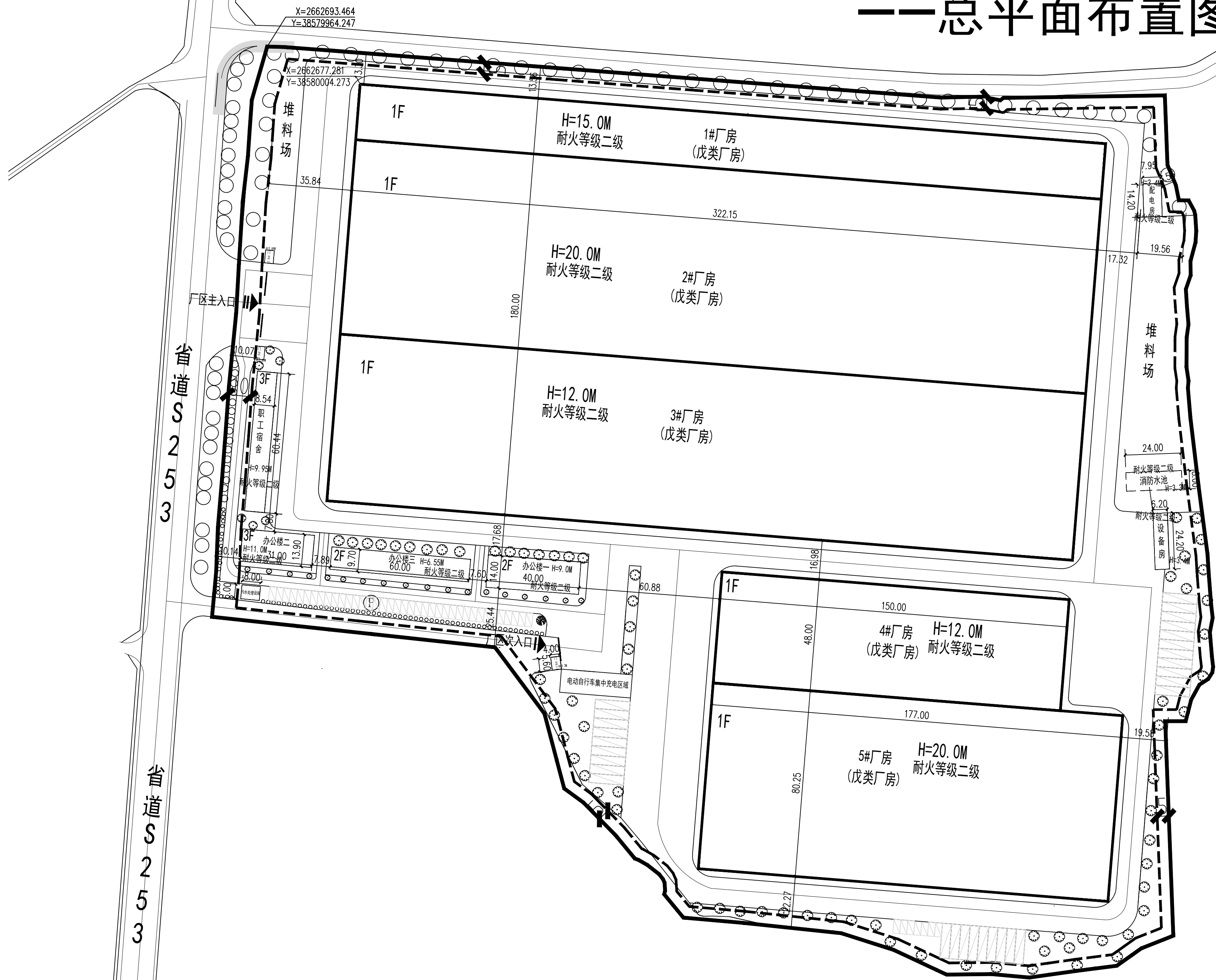
总平面图 1:800
